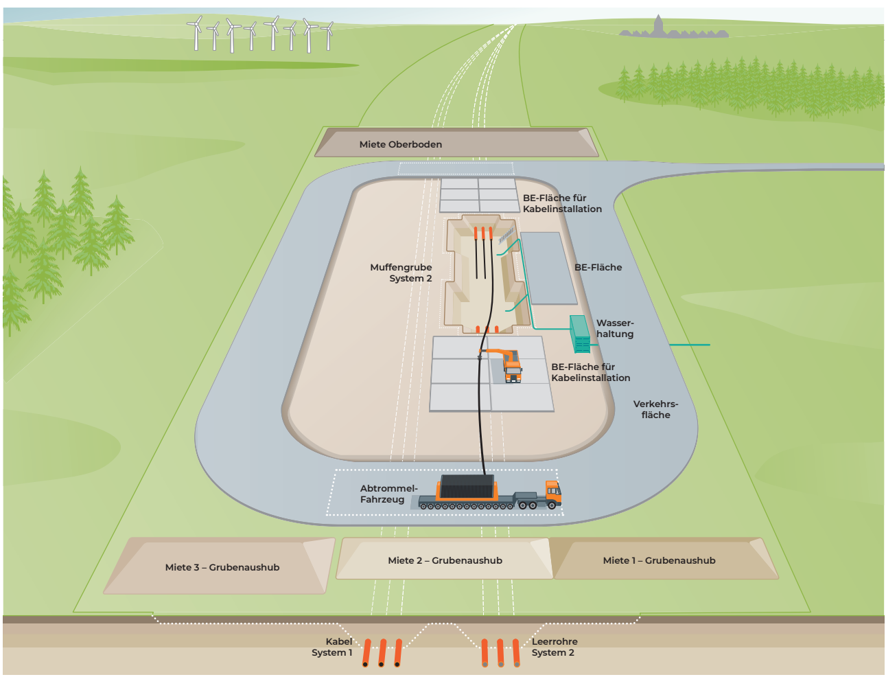
Anlieferung und Einzug der Kabel für System 2
