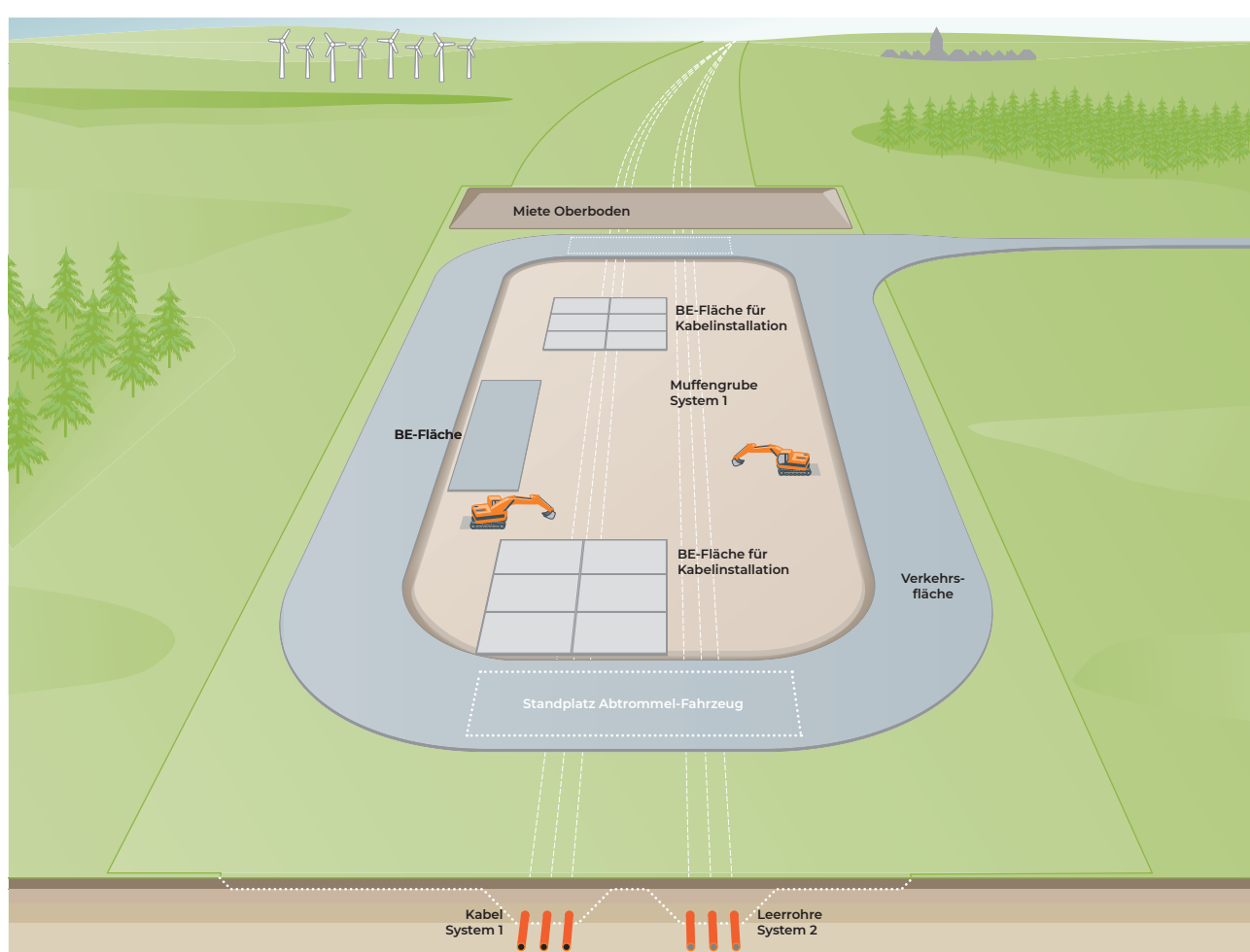
Verfüllen der Muffengrube für System 1
