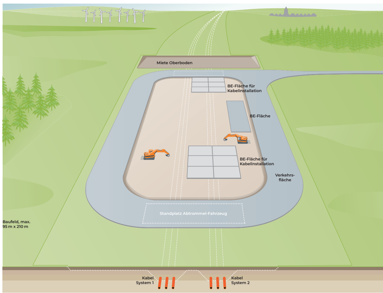
Verfüllen der Muffengrube für System 2
