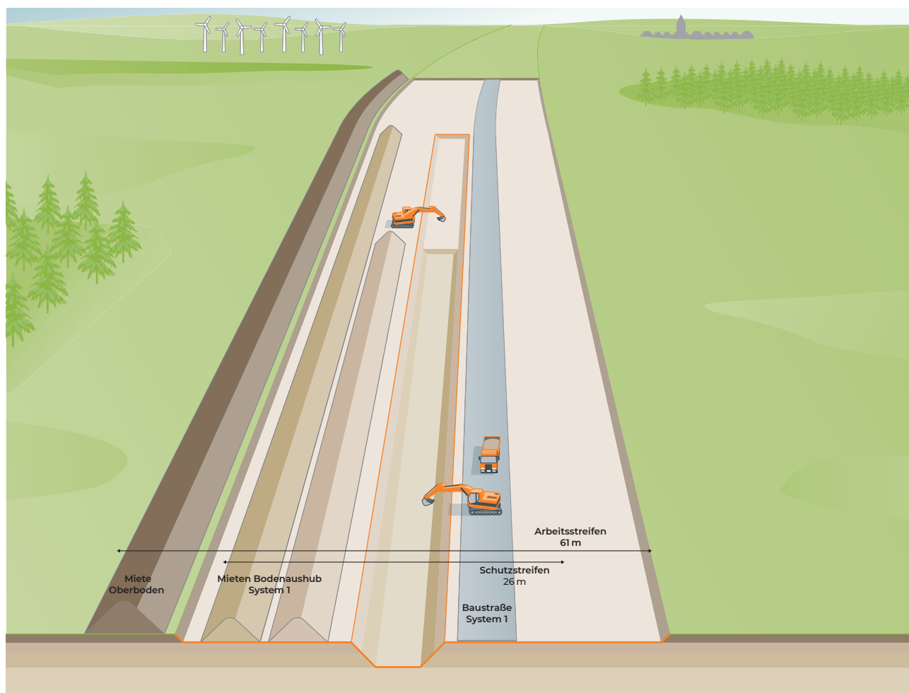
Bodenaushub nach Erdschichten für System 1
