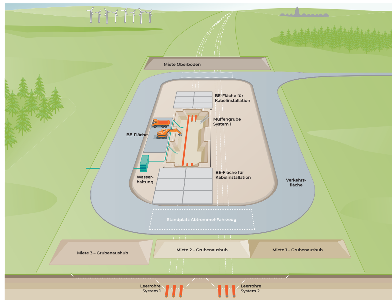
Ausheben der Muffengrube für System 1 und Herausschneiden der Leerrohre im Bereich der Muffengrube
