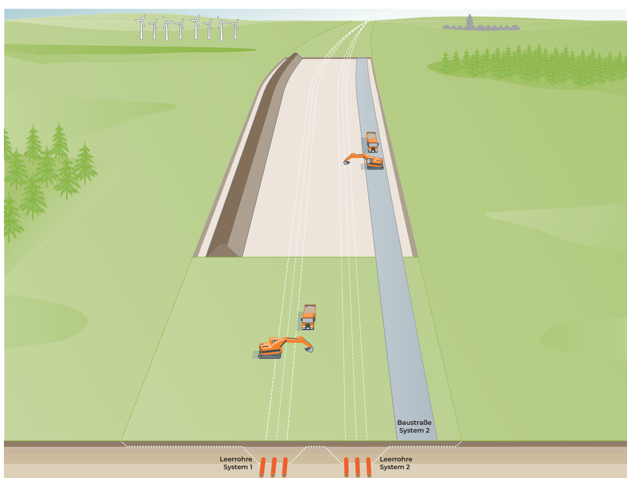
Wiederverfüllung des Oberbodens
