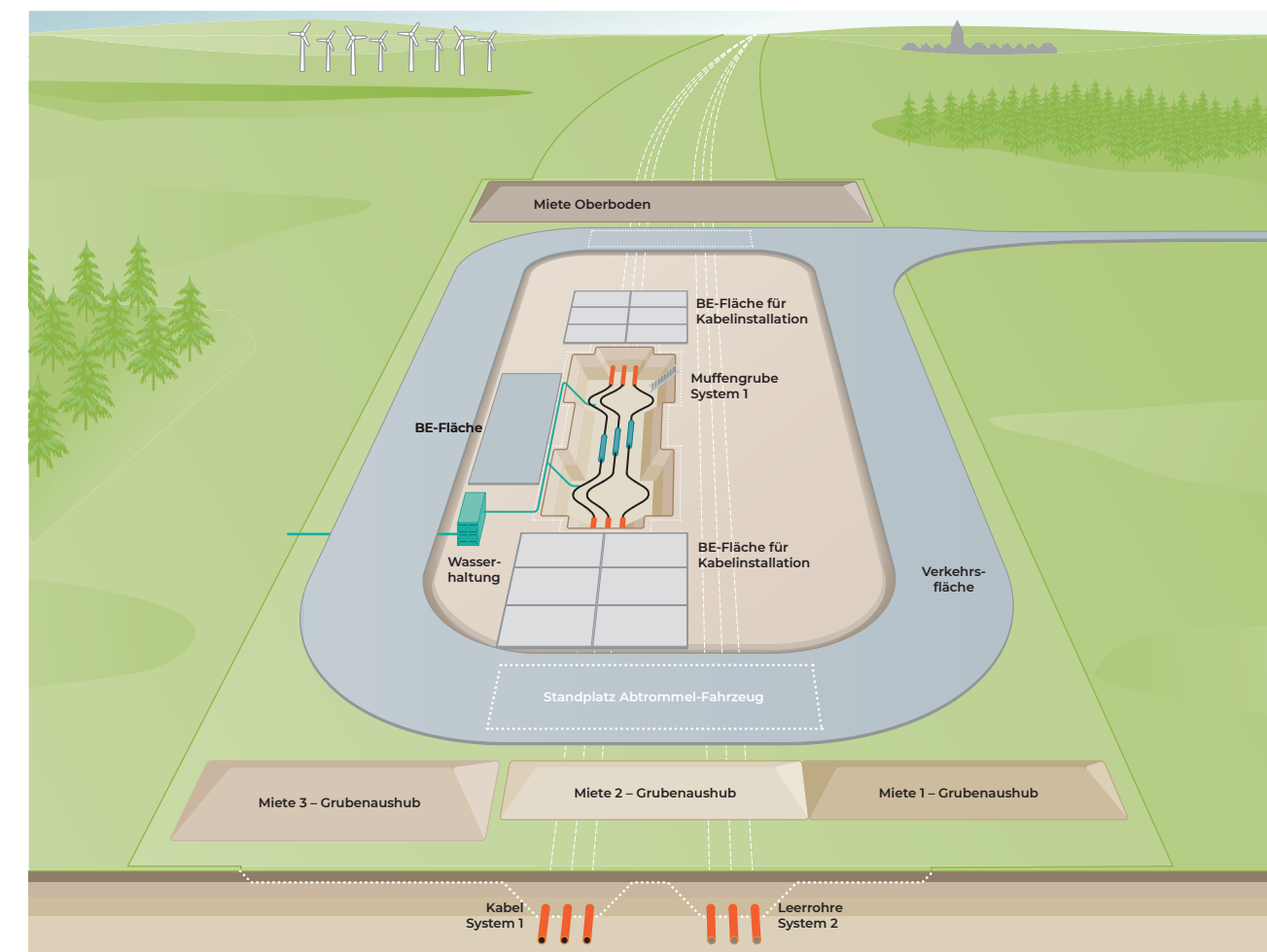
Rückbau der Container, die Kabel liegen verbunden in der Muffengrube
