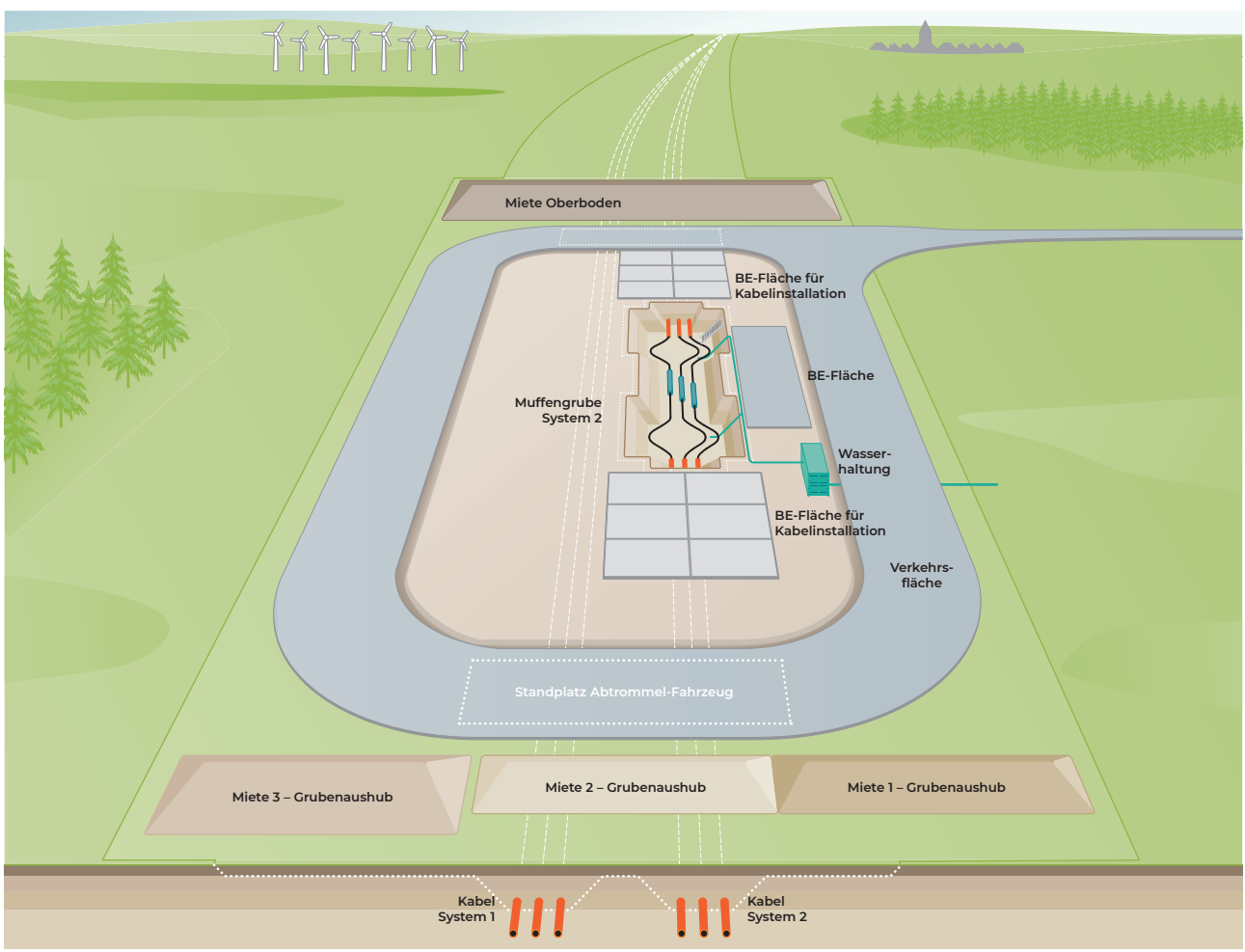
Rückbau der Container, die Kabel liegen verbunden in der Muffengrube
