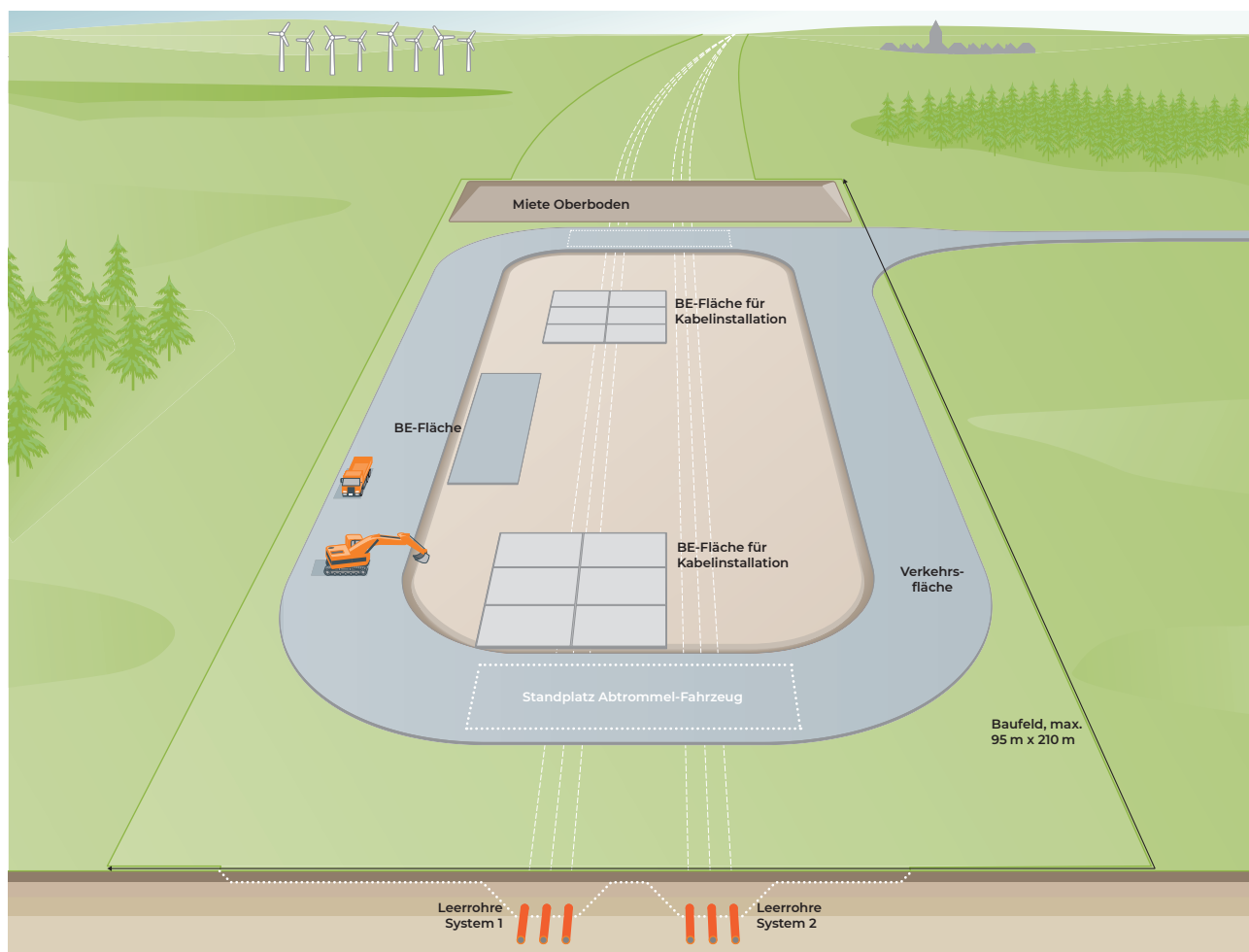
Errichtung der Baustraße und Befestigung der Baueinrichtungsflächen für System 1
