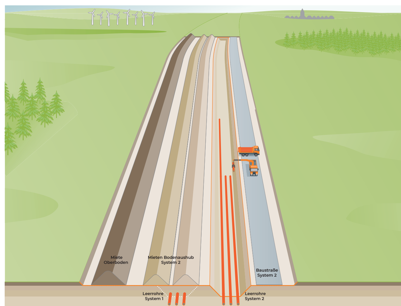
Verlegen der Leerrohre für System 2
