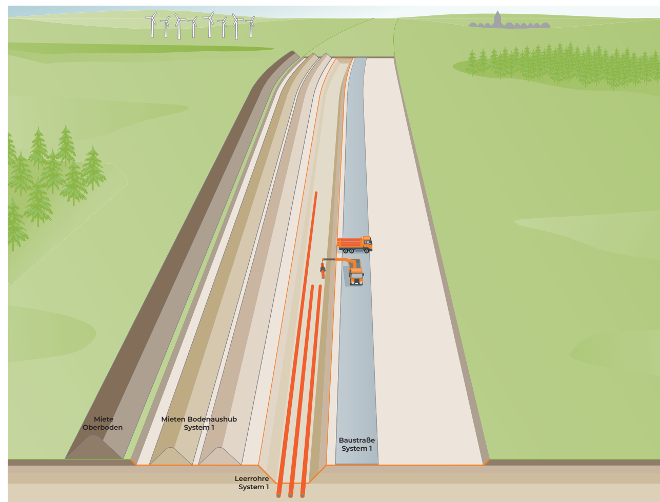
Verlegen der Leerrohre für System 1
