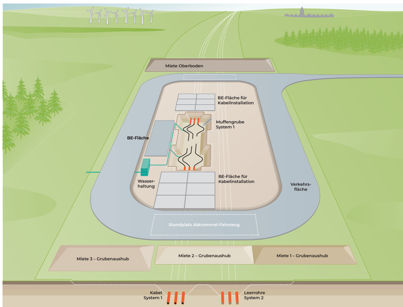
Kabel werden in Kurvenform gelegt um Reserve für Reparaturfall zu haben
