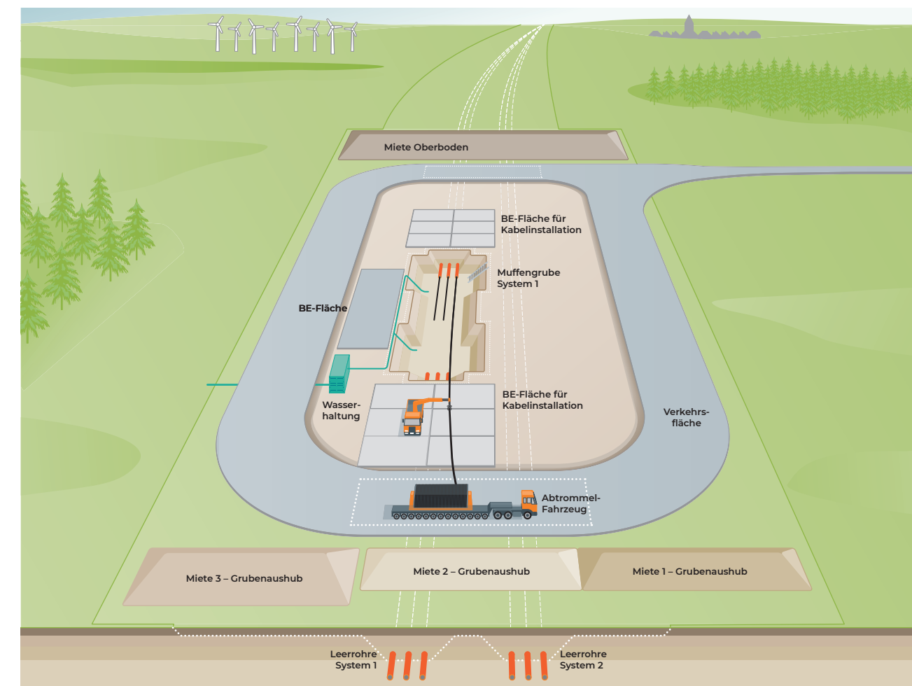
Anlieferung und Einzug der Kabel für System 1
