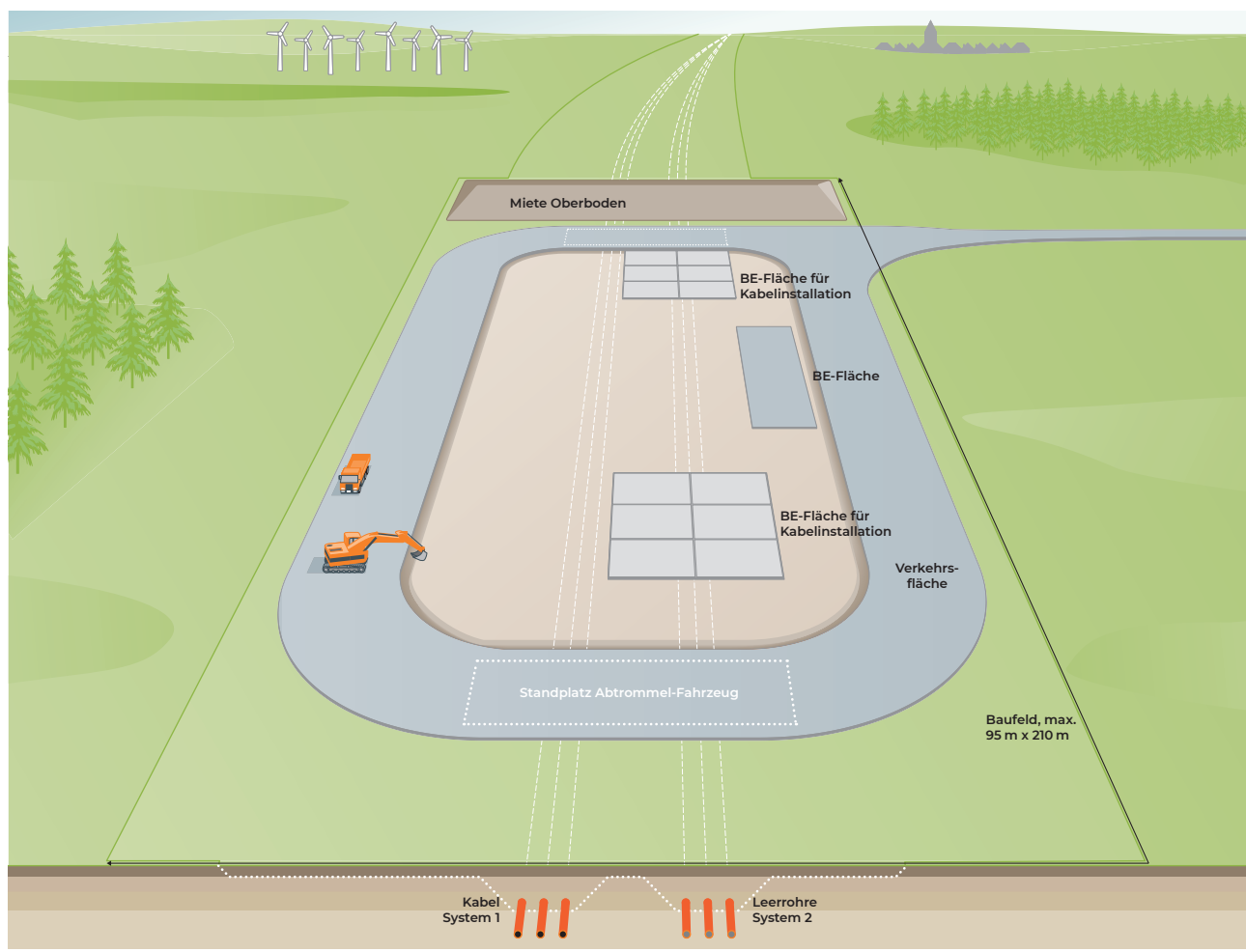
Errichtung der Baustraße und Befestigung der Baueinrichtungsflächen für System 2
