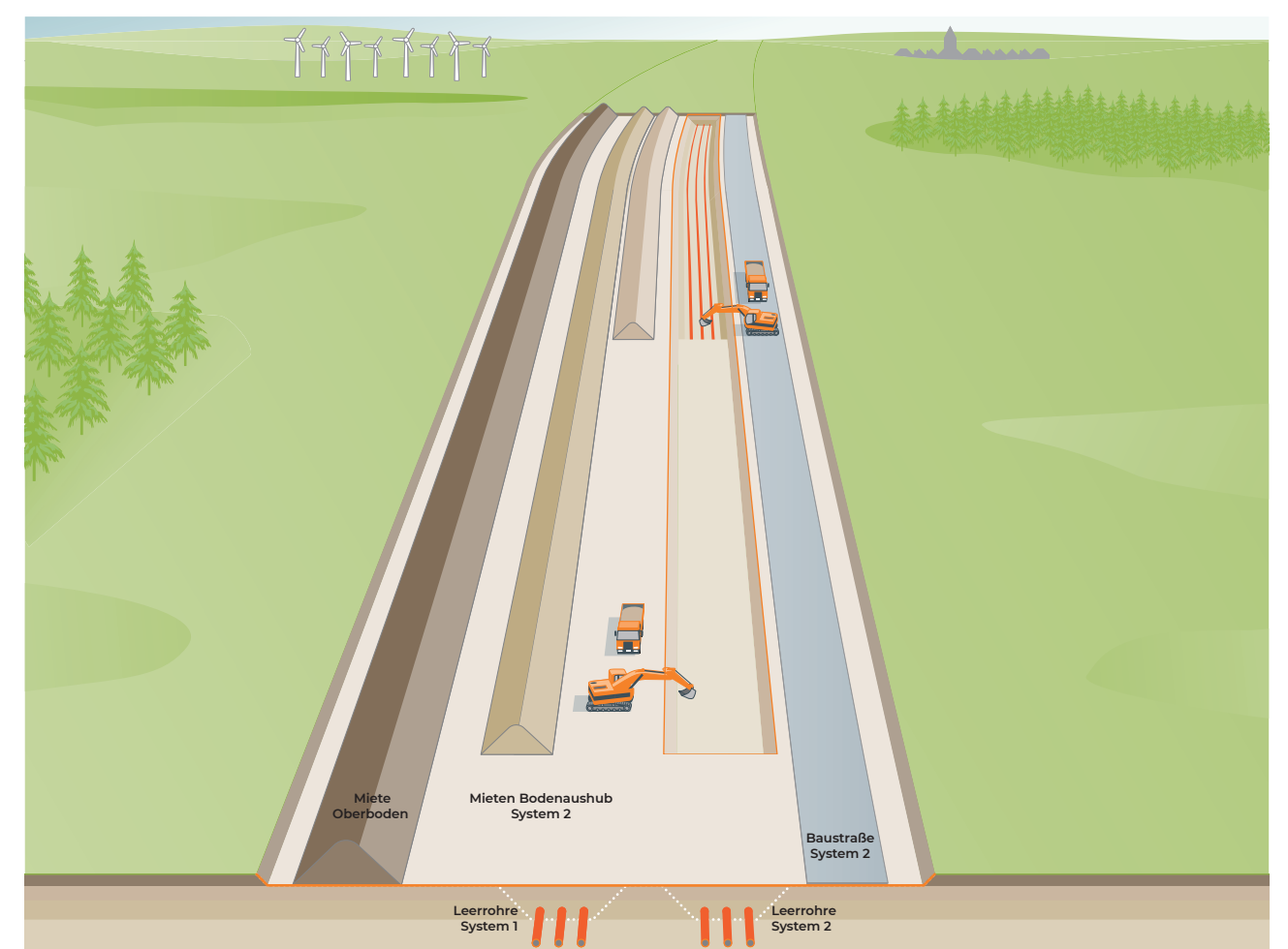
Verfüllen nach Erdschichten für System 2
