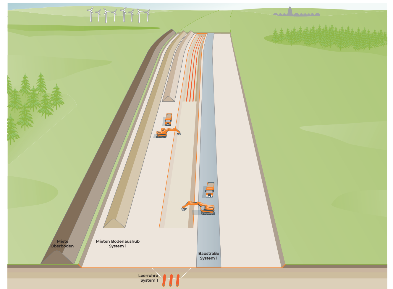
Verfüllen nach Erdschichten für System 1
