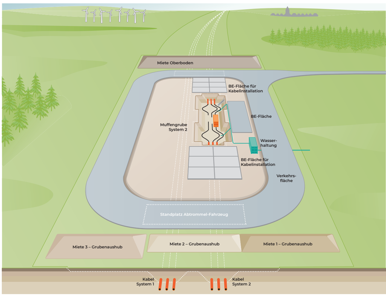
Die Installation der Muffen erfolgt in speziellen Containern
