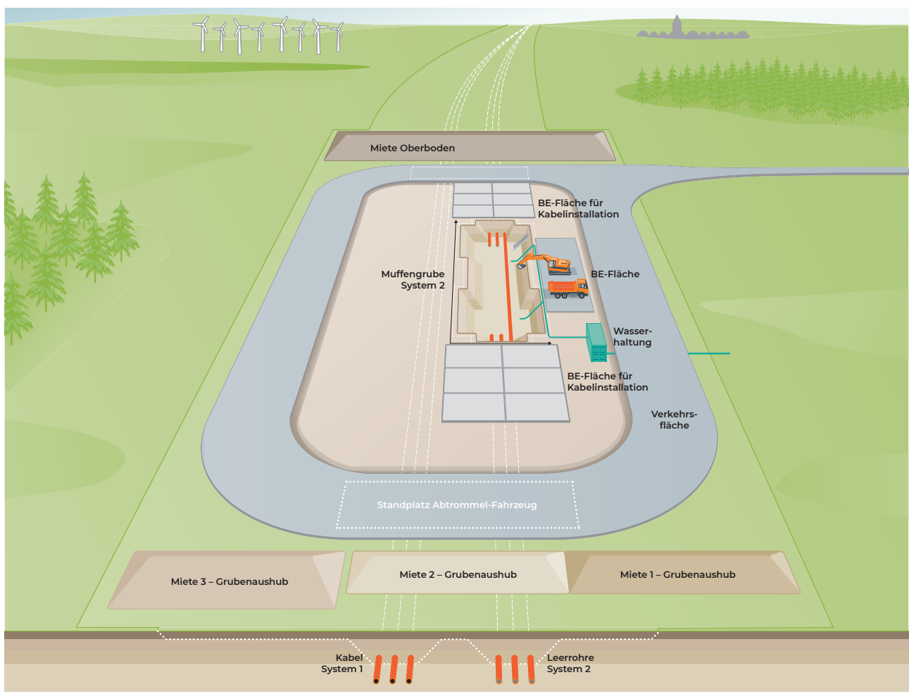
Ausheben der Muffengrube für System 2 und Herausschneiden der Leerrohre im Bereich der Muffengrube
