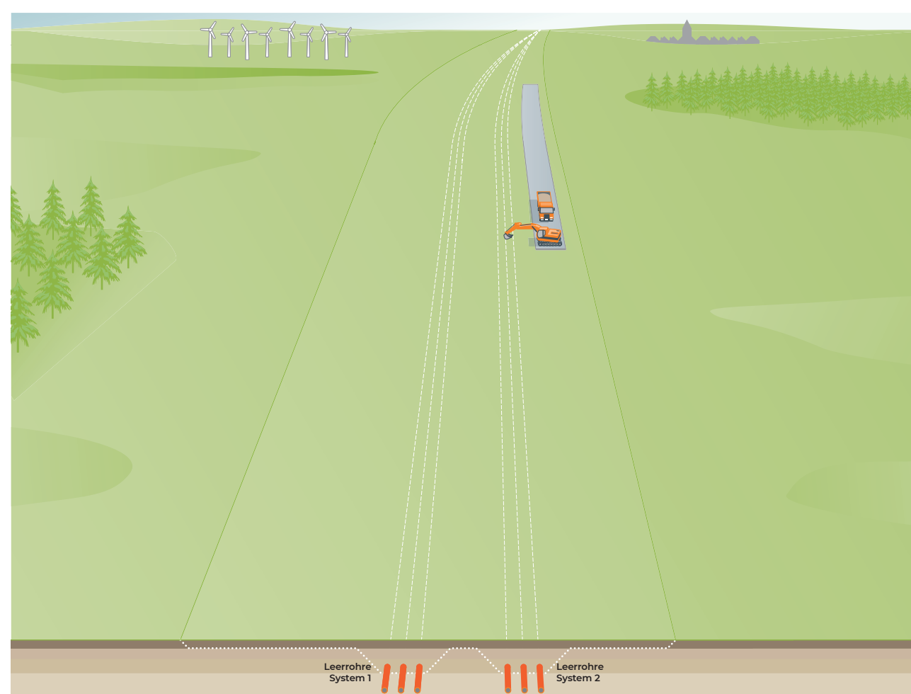
Rückbau der Baustraße
