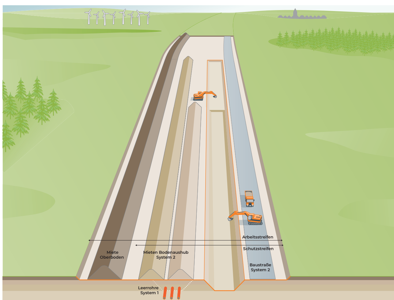
Bodenaushub nach Erdschichten für System 2
